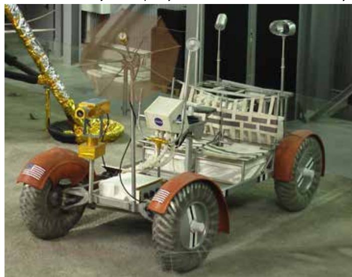
Replika měsíčního džípu LRV (Lunar Roving Vehicle) v Technickém muzeu ve Speyeru
